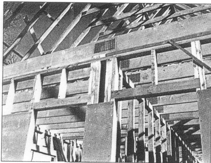
A földémszerkezet kialakítása
