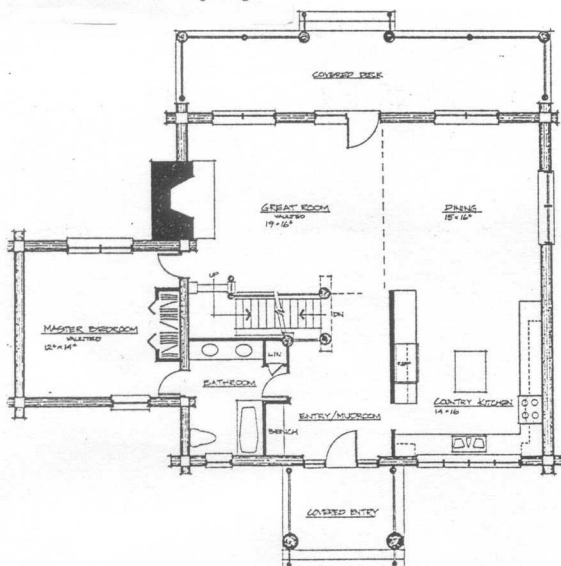
Földszinti alaprajz
