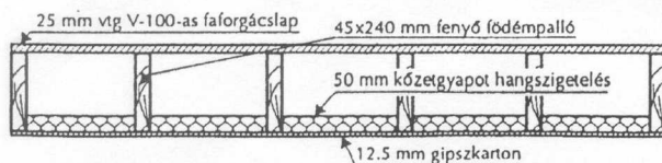
A földémszerkezet kialakítása
