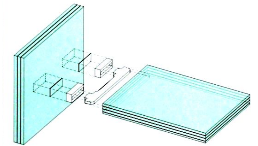
23. ábra Tiszta üveg szerkezetű lépcső fokainak rögzítése. Sedak-Seele, Glasstec 2006.
