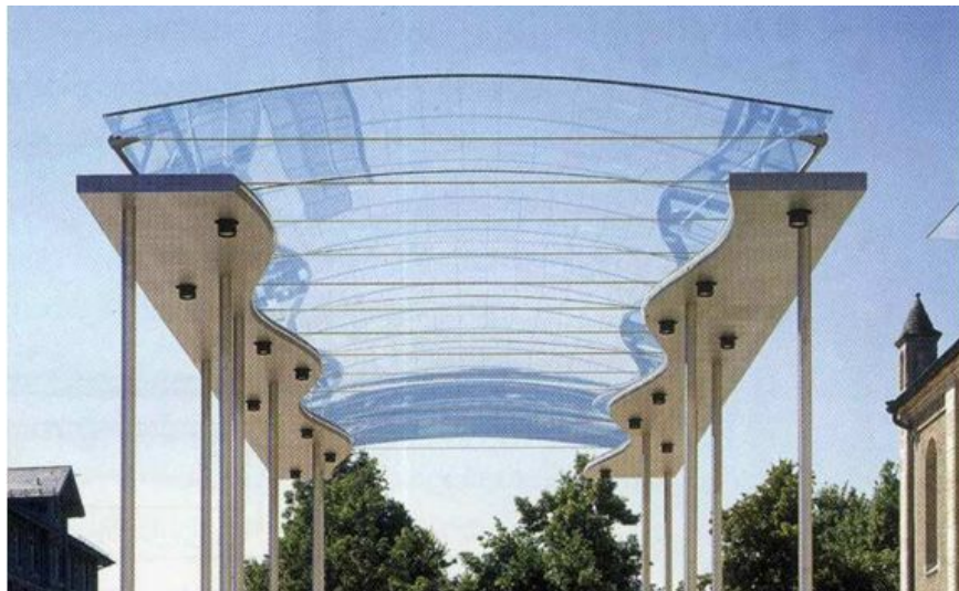
11. ábra Aláfeszített üveg donga – szabadalommal védett német szerkezeti megoldás
