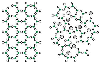
1. ábra A homok (a bal oldalon) és a nátronüveg (jobb oldal) molekuláris felépítése
