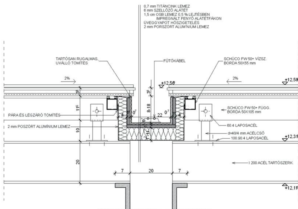
18. ábra Az Alkotás Point irodaház átriumának vízelvezetése
