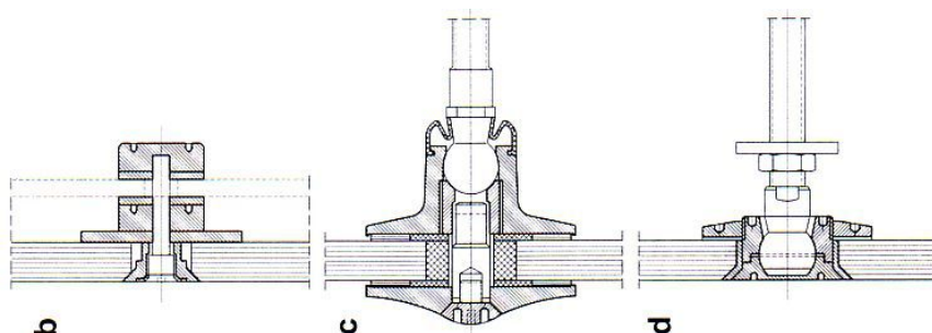
19. ábra A pontmegfogó szerelvények erőtani szempontból különböző kialakítása: b.) merev, c.) külső csuklós, d.) belső csuklós
