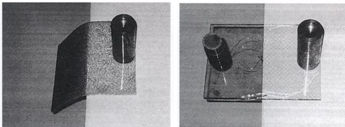
7. ábra A maradó szilárdság szemléltetése. A bal oldali üvegtábla két edzett üvegből, a jobb oldali két hőerősített üvegből van ragasztva
