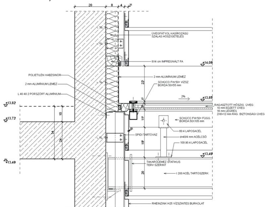
17. ábra Az Alkotás Point irodaház átriumának falcsatlakozása. (Építész Cságoly Ferenc, Keller Ferenc és Hönich Richárd, épületszerkezeti tervező Becker Gábor)
