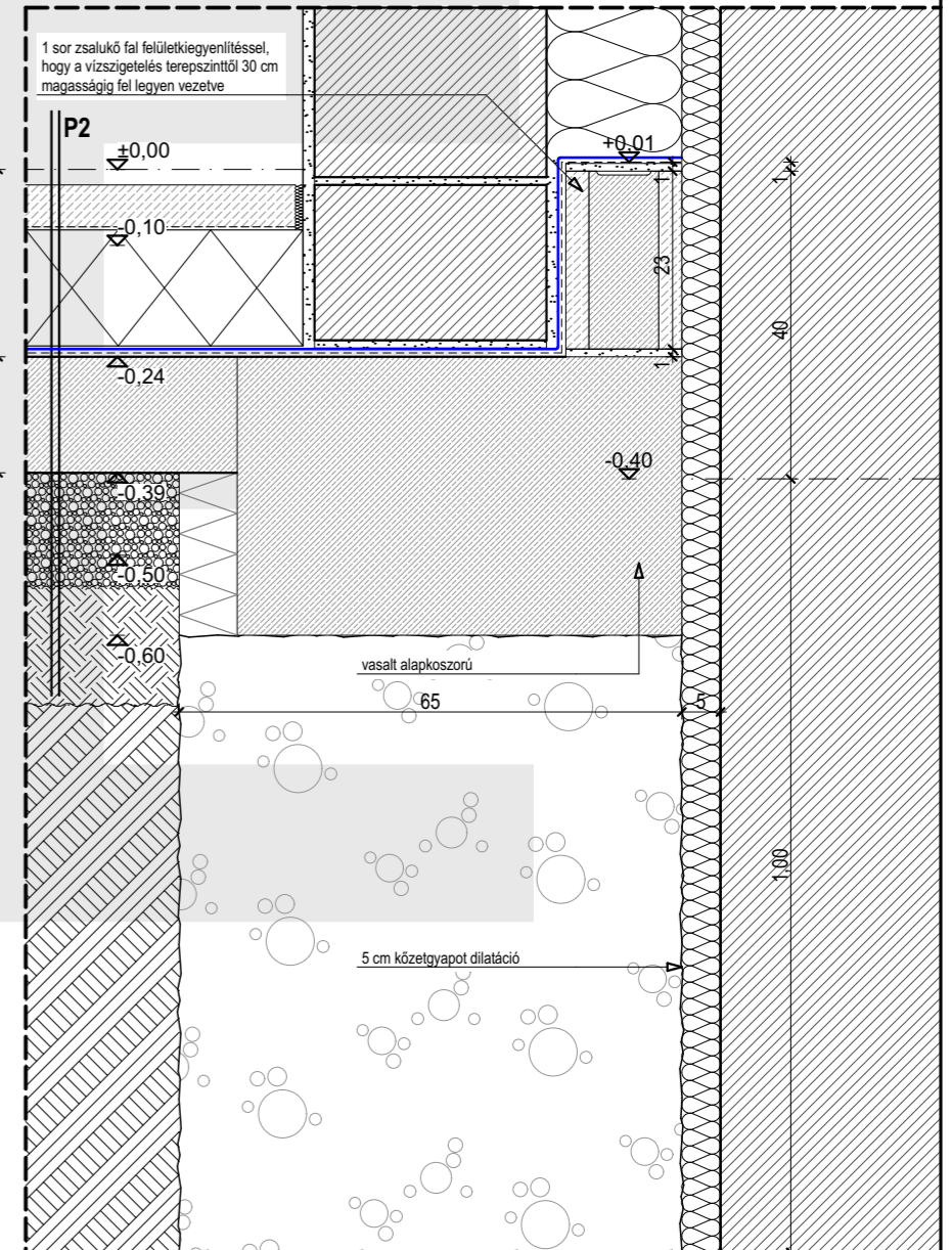
CSP5 - Szomszéd csatlakozás
