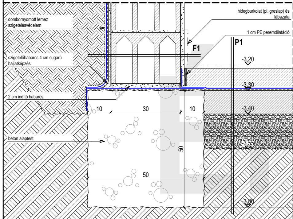
CSP2 - Szélső főfal alapozása
