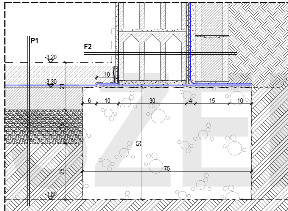
CSP4 - Szintváltás alsó részlete
