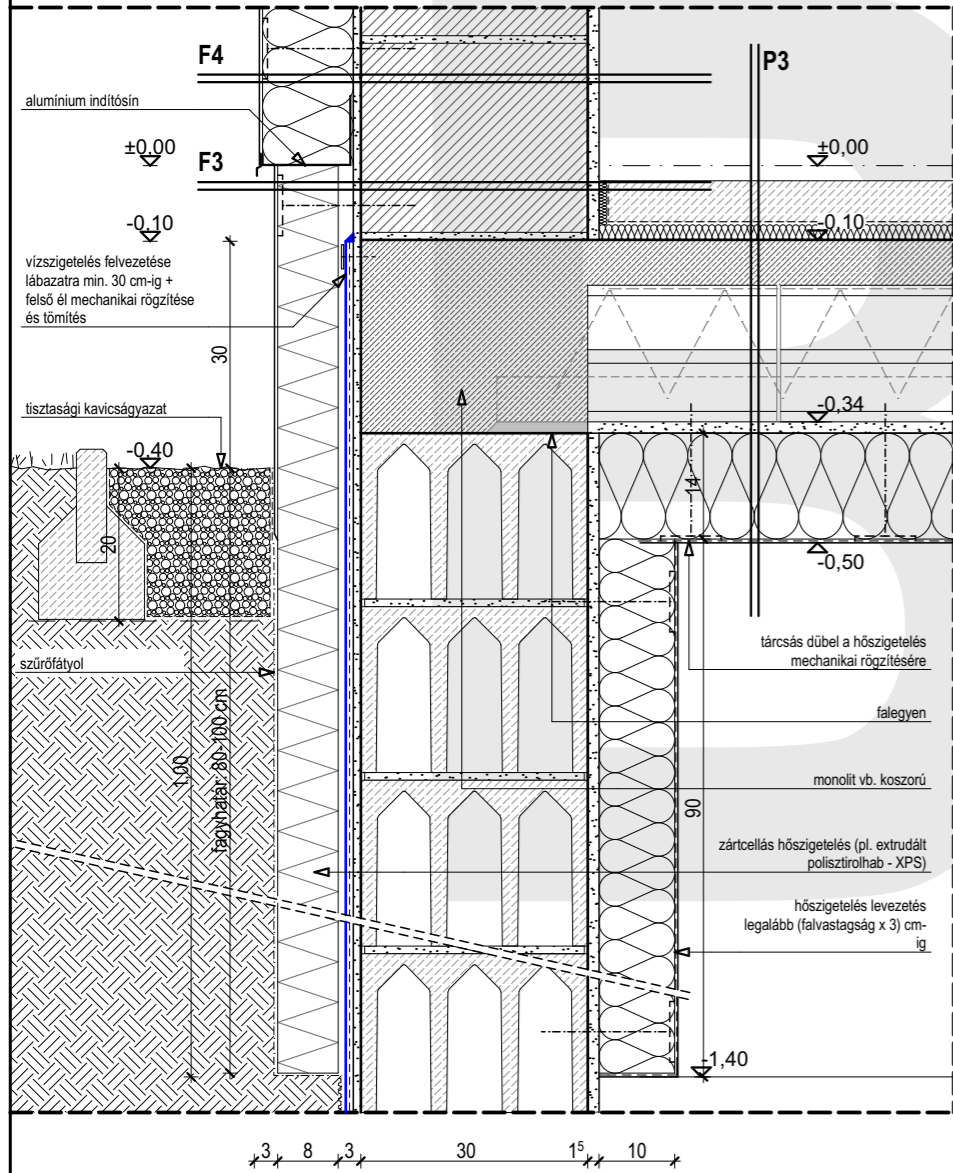
CSP2 - Szélső főfal alapozása
