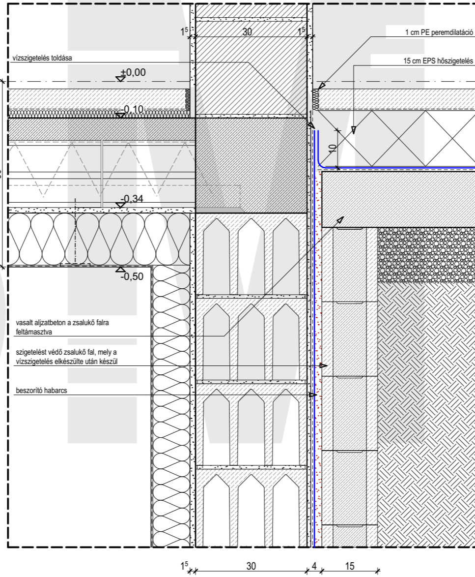
CSP4 - Szintváltás alsó részlete
