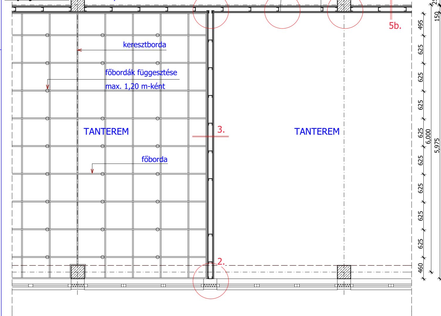
Alaprajz M=1:50
