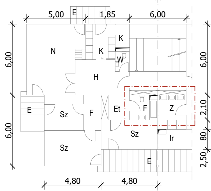
Alaprajzi vázlat M=1:200
