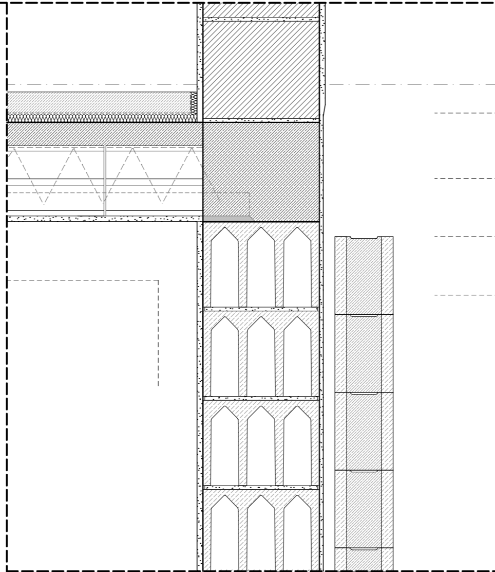
Szintváltás felső részlete
