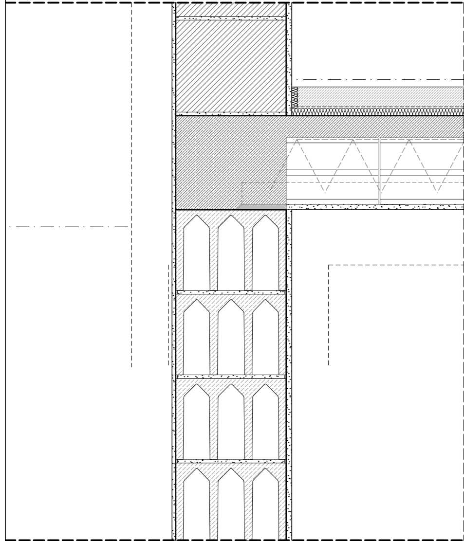
Lábazat alapincézett épületrész esetén
