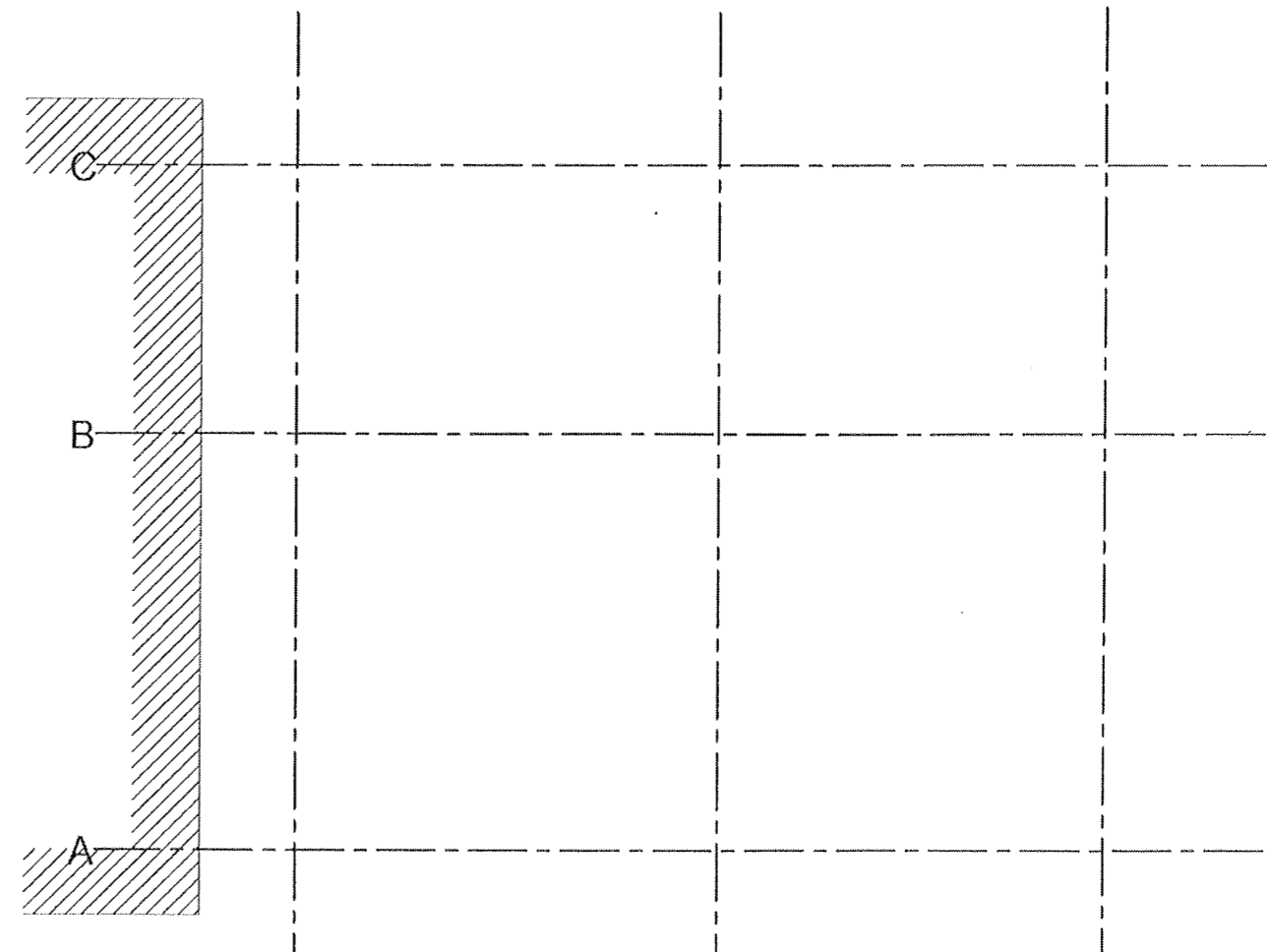
VÍZSZINTES SÍKKOORDINÁCIÓ M 1:25
