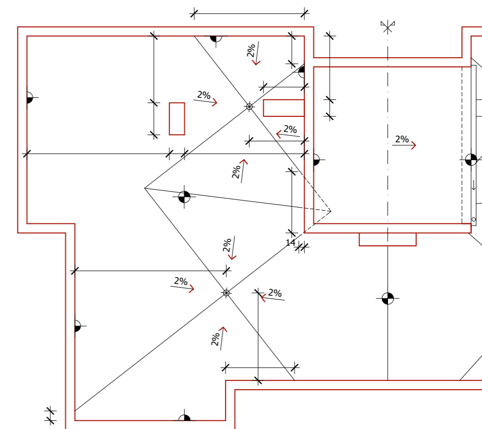
derékszögű szerkesztés - több lefolyó beépítése
