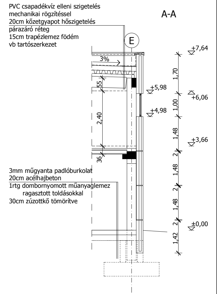
Homlokzat nézete és A-A részmetset m= 1:100
