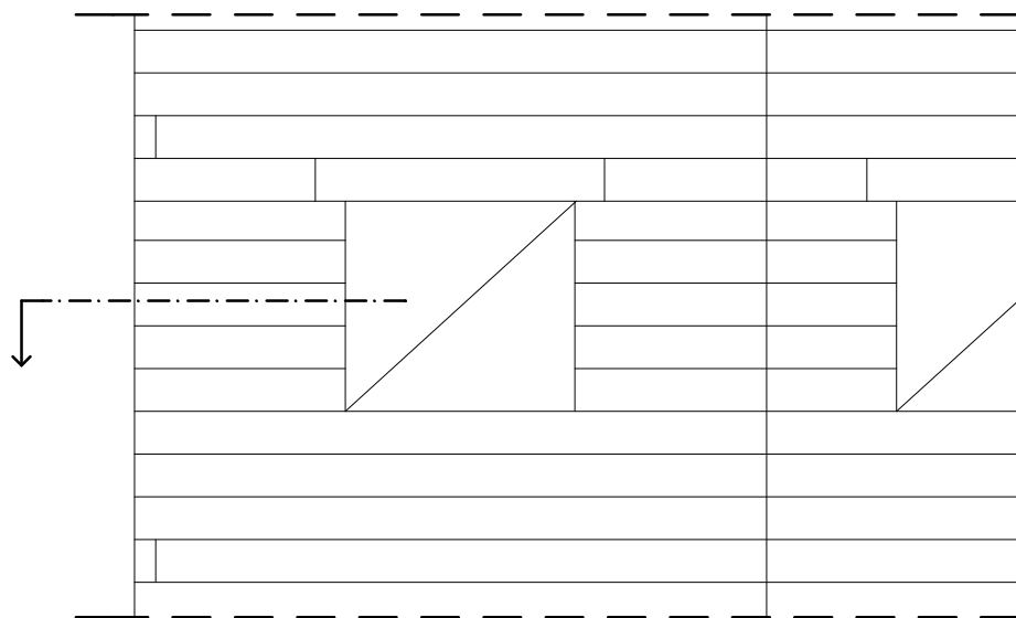
FALSZAKASZ ALAPRAJZA, m = 1:25
