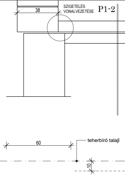
LÁBAZAT KIALAKÍTÁSÁNAK CSOMÓPONTJA, ( 2-es Vari.) 30 cm-nél kisebb kiemelés esetén
