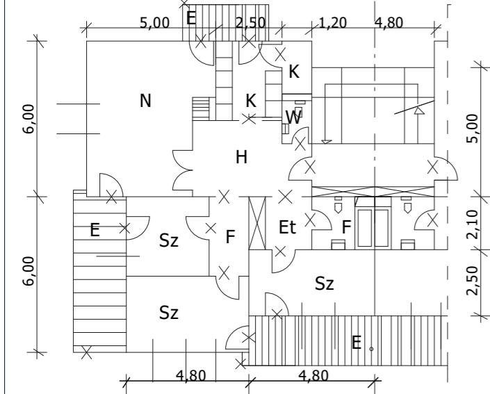
Alaprajz M=1:100
