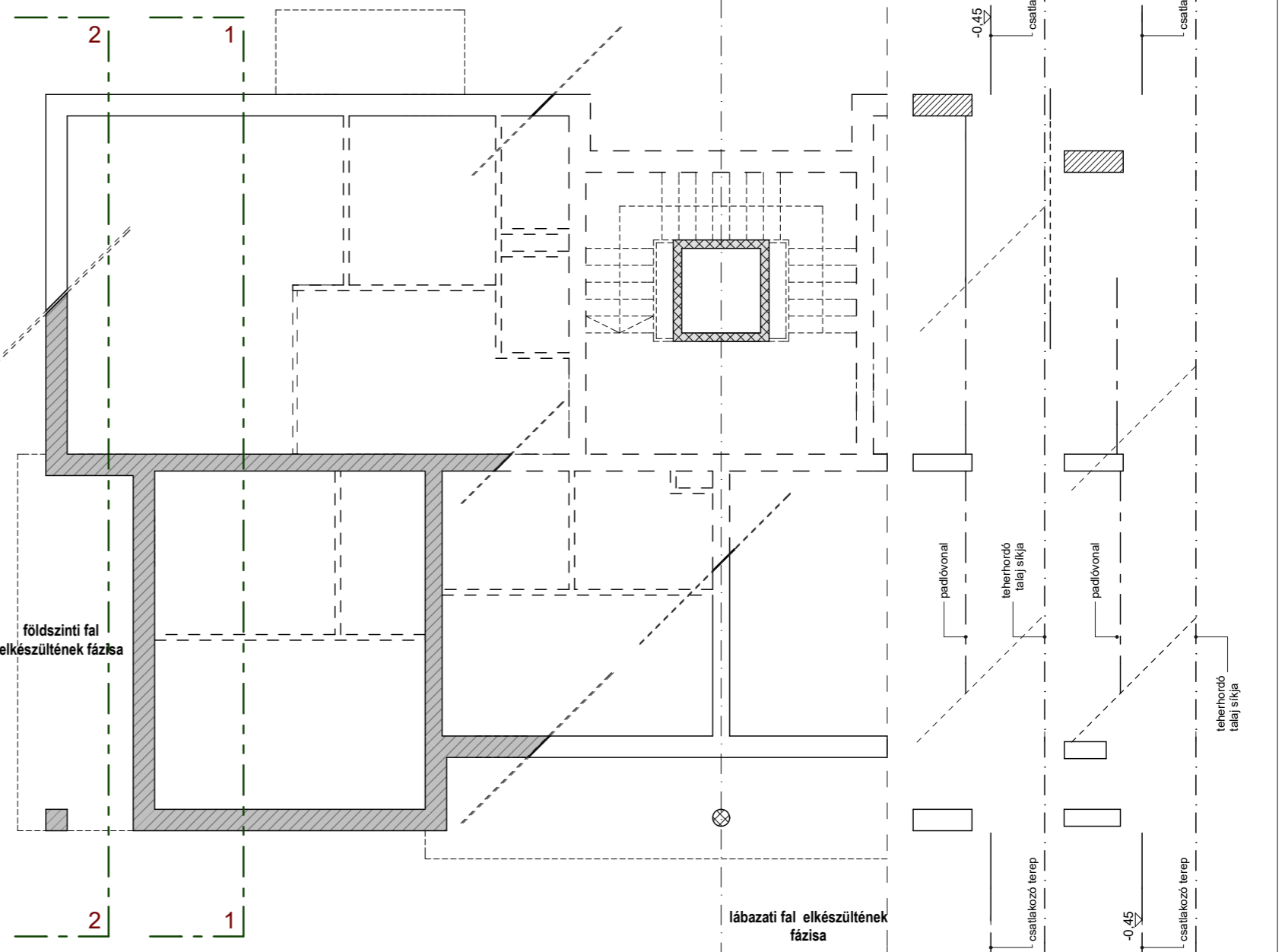
Alapozási Terv M=1:100 lábati fal elkészültének fázisa
