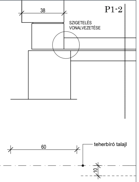
LÁBAZAT KIALAKÍTÁSÁNAK CSOMÓPONTJA, ( 2-es Vari.) 30 cm-nél kisebb kiemelés esetén
