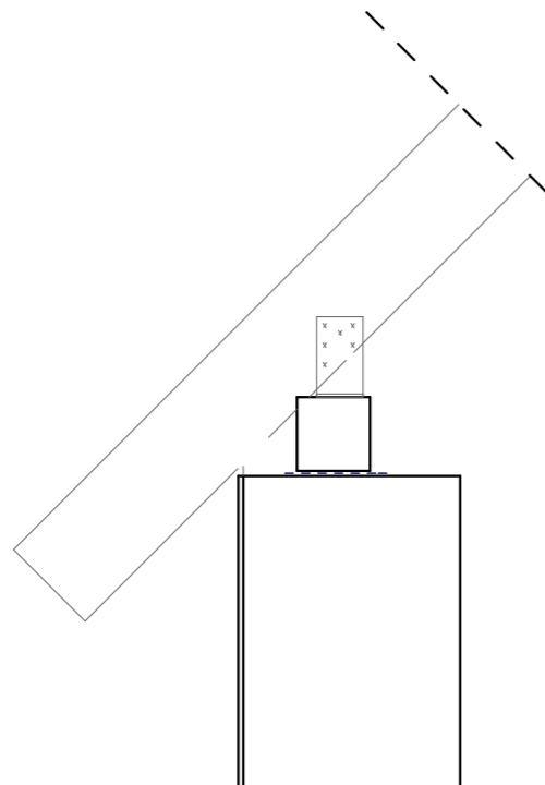
CSOMÓPONTOK KÖRÜLHORNYOLT CSERÉP ALKALMAZÁSÁVAL- ERESZKIALAKÍTÁS
