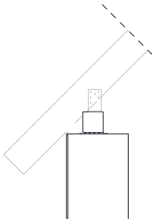
CSOMÓPONTOK KETTŐS HÓDFARKÚ CSERÉP ALKALMAZÁSÁVAL- ERESZKÉPZÉS
