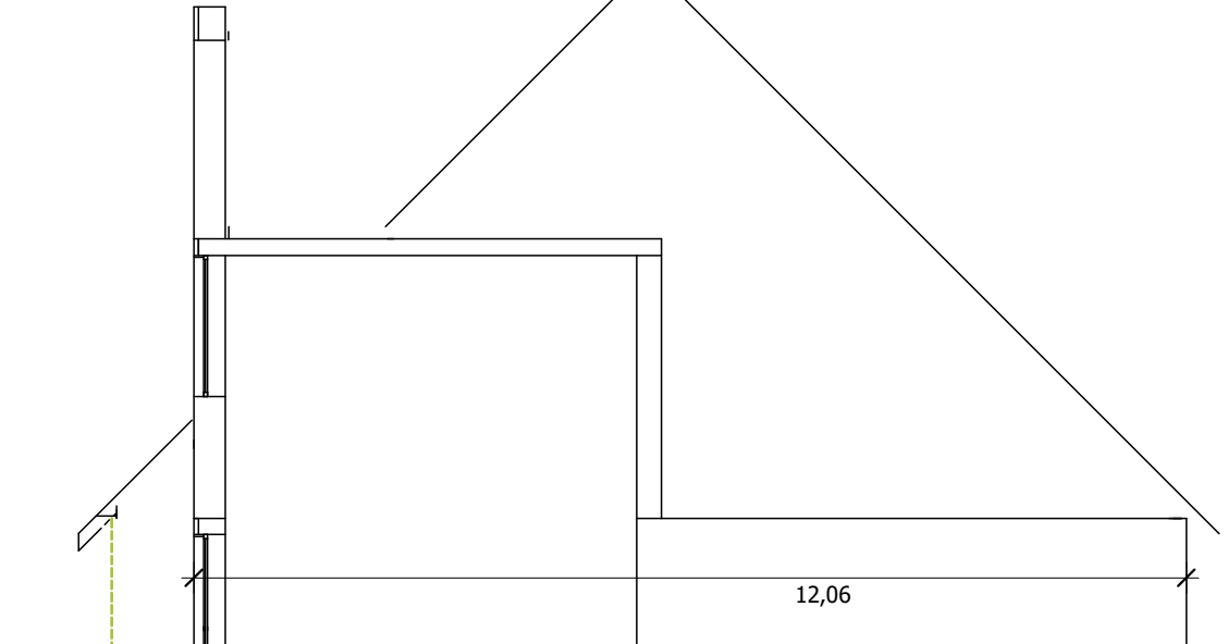
4. Metszet M=1:100
