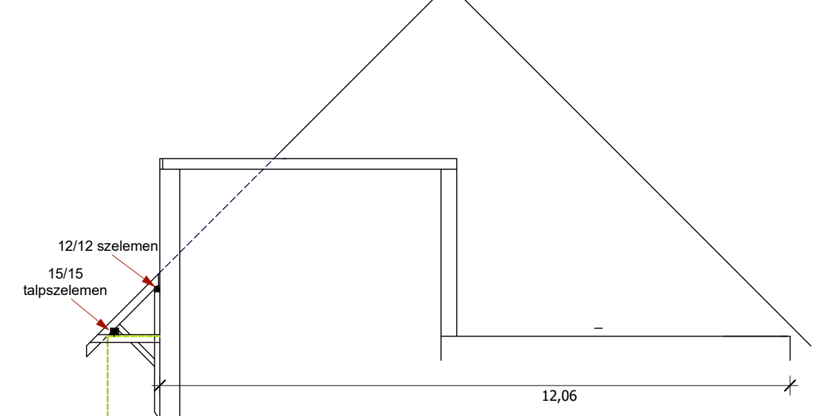
3. Metszet M=1:100
