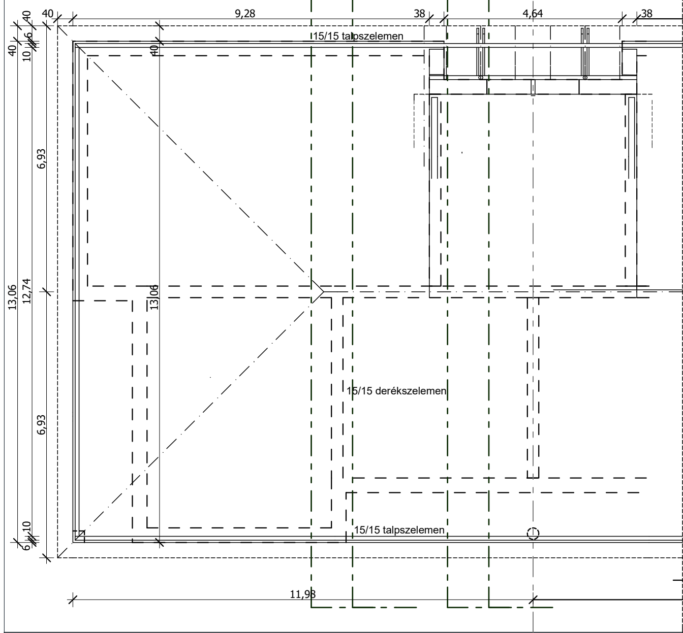
Tetőszerkezeti alaprajz M=1:100
