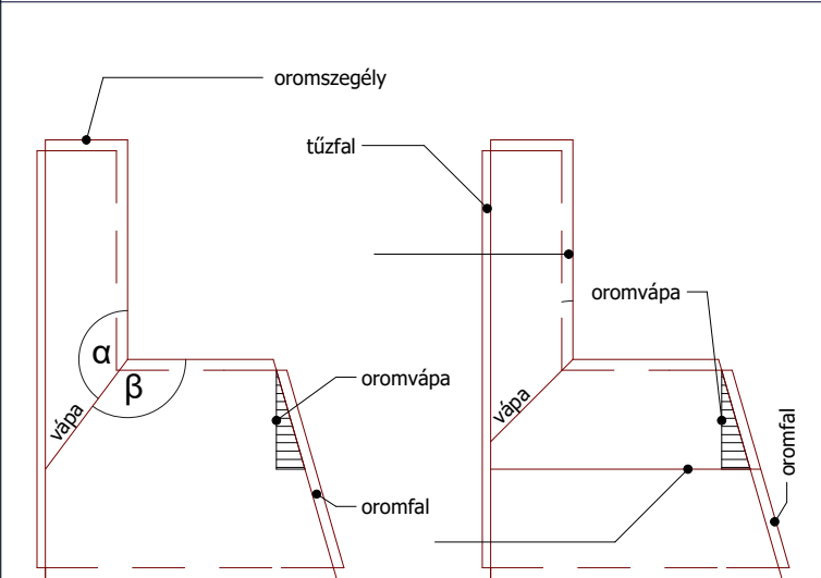
Alaprajzi és homlokzati séma
