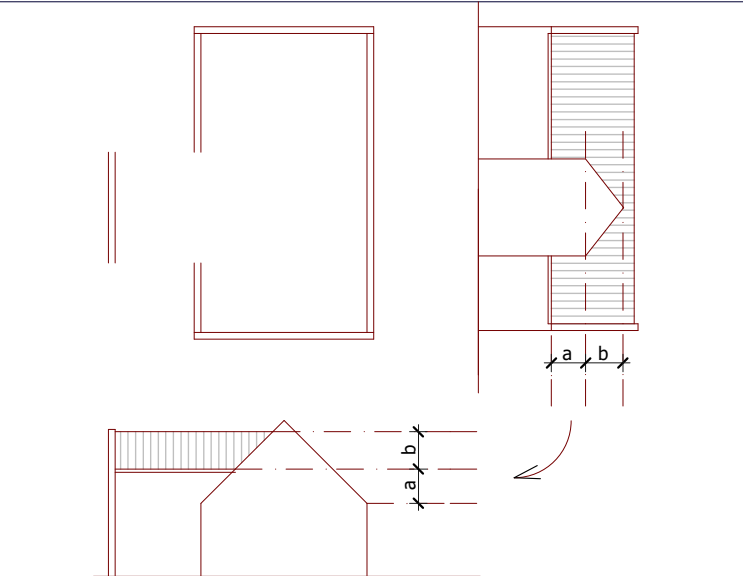
Összemetszések eltérő magasságú párkányok esetén
