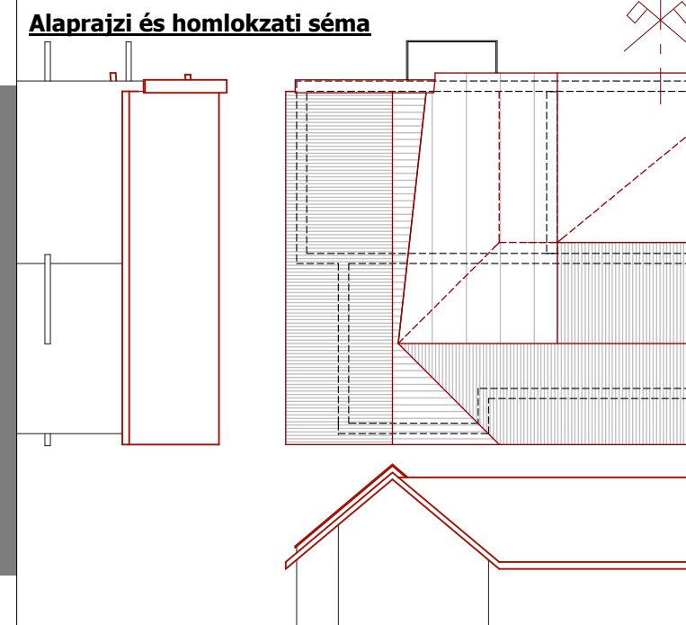
Tömegvázlat
