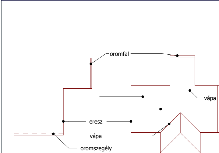
Összemetsződés szerkesztési sémája
